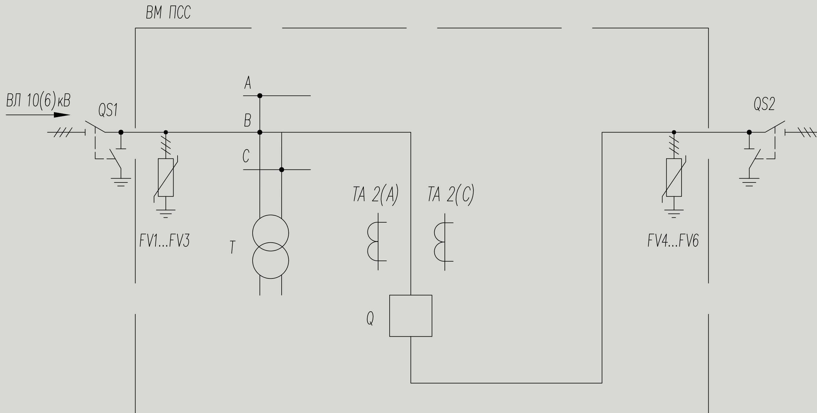
Рисунок 2—Схема главных цепей ПСС-1 в сети с односторонним питанием
