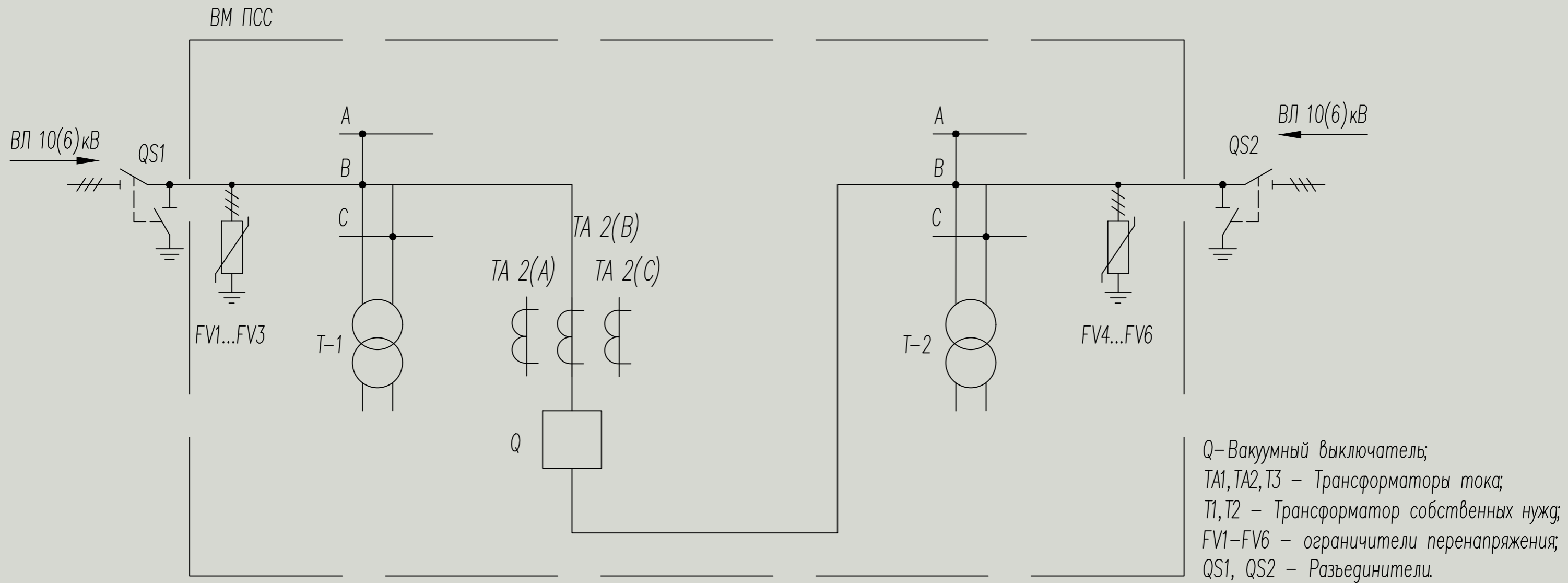
Рисунок 3 – Схема главных цепей ПСС-2 в сети с двусторонним питанием
